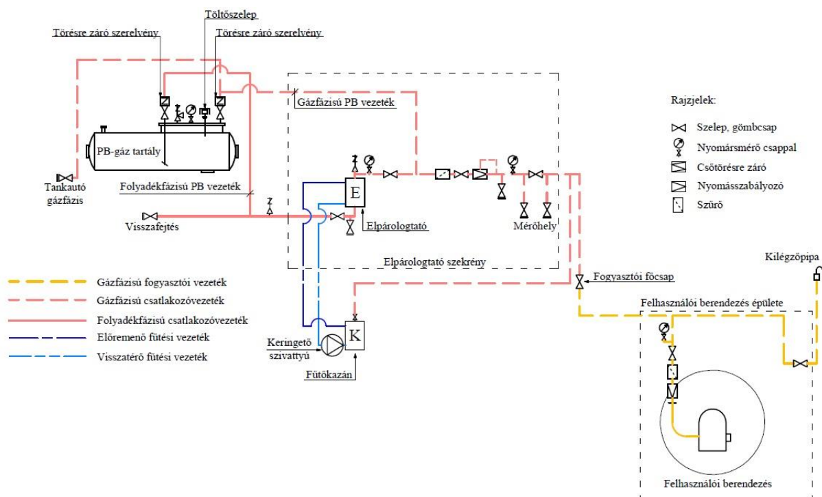
7. ábra: A csatlakozóvezeték és fogyasztói vezeték határai elpárolgató PB-gáz felhasználói berendezés esetén
