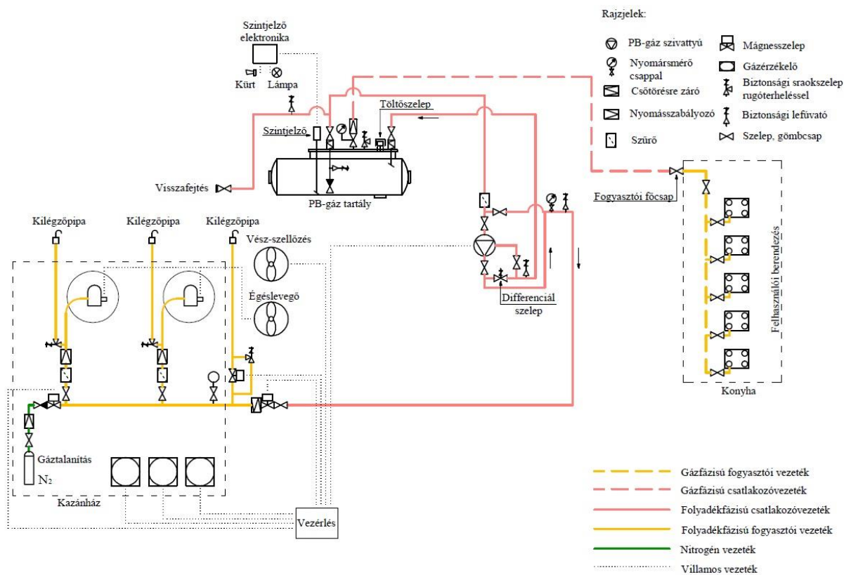
8. ábra: Csatlakozóvezeték és a fogyasztói vezeték határai szivattyús és egyszerű PB-gáz felhasználói berendezés esetén
