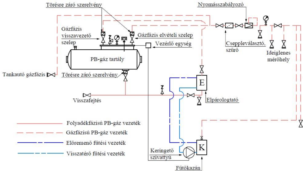
3. ábra: Tartályra dolgozó elpárolgató beépítése
