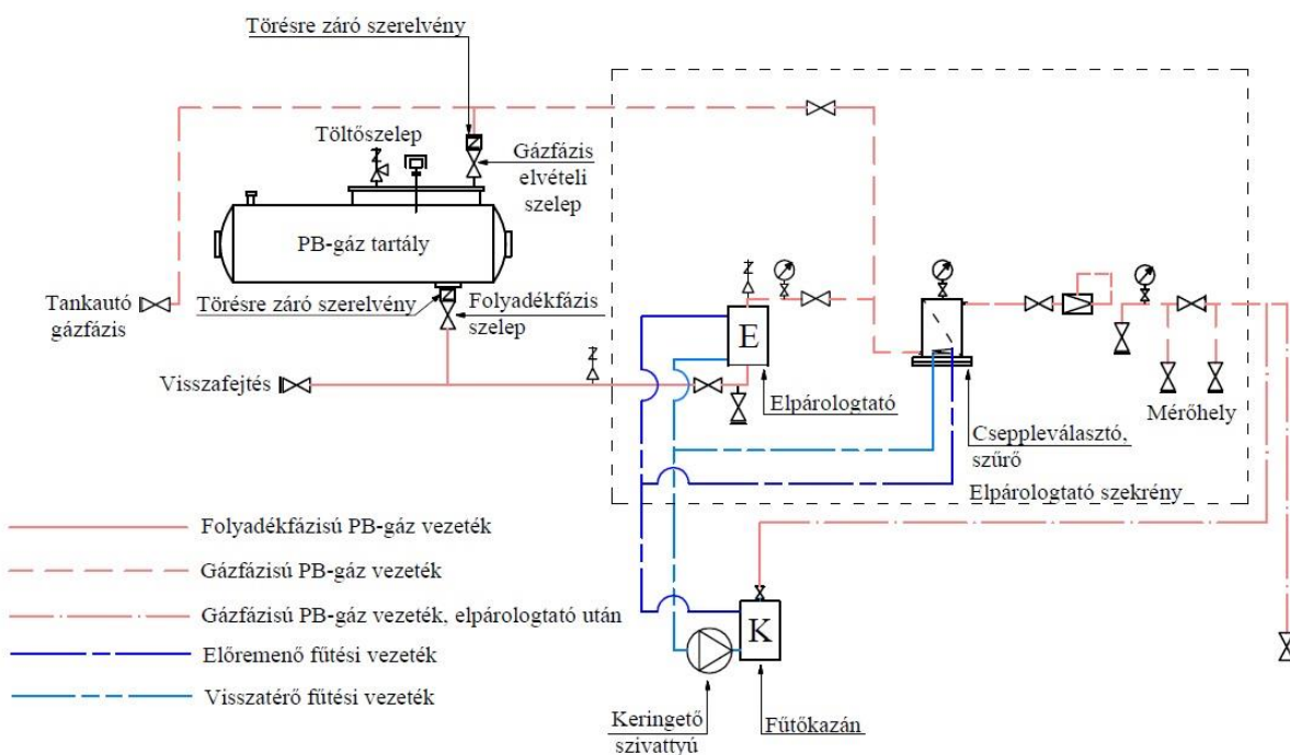
4. ábra Csatlakozóvezetékre dolgozó szekrényes elpárolgató berendezés beépítése
