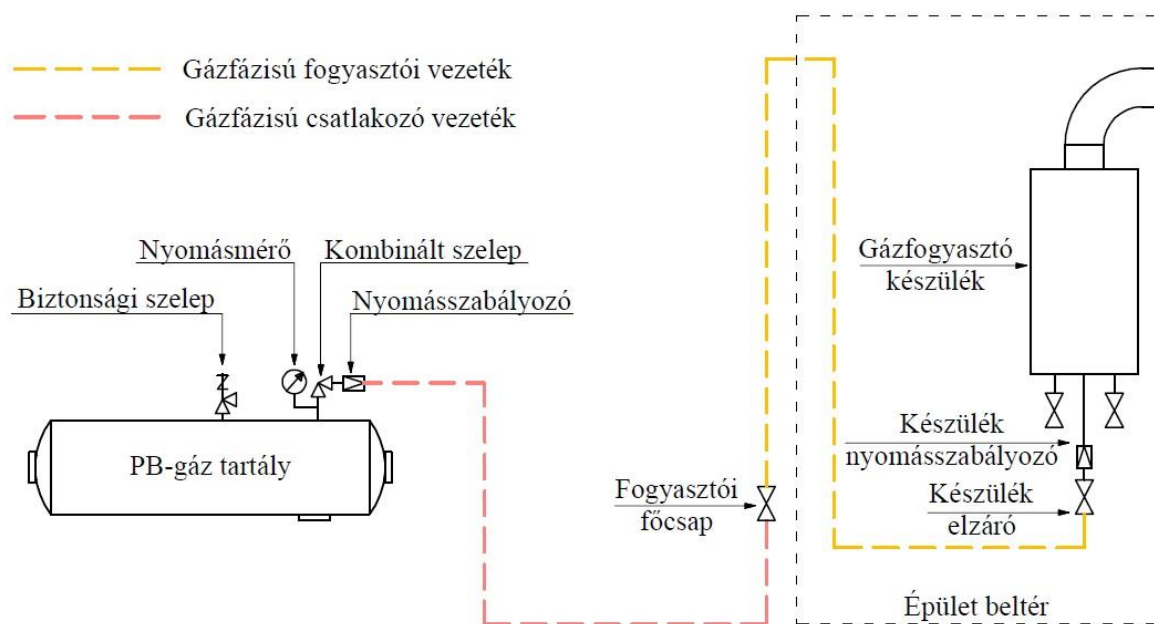
6. ábra: A csatlakozóvezeték és a fogyasztói vezeték egyszerű (elpárolgató nélküli) PB-gáz felhasználói berendezés esetén
