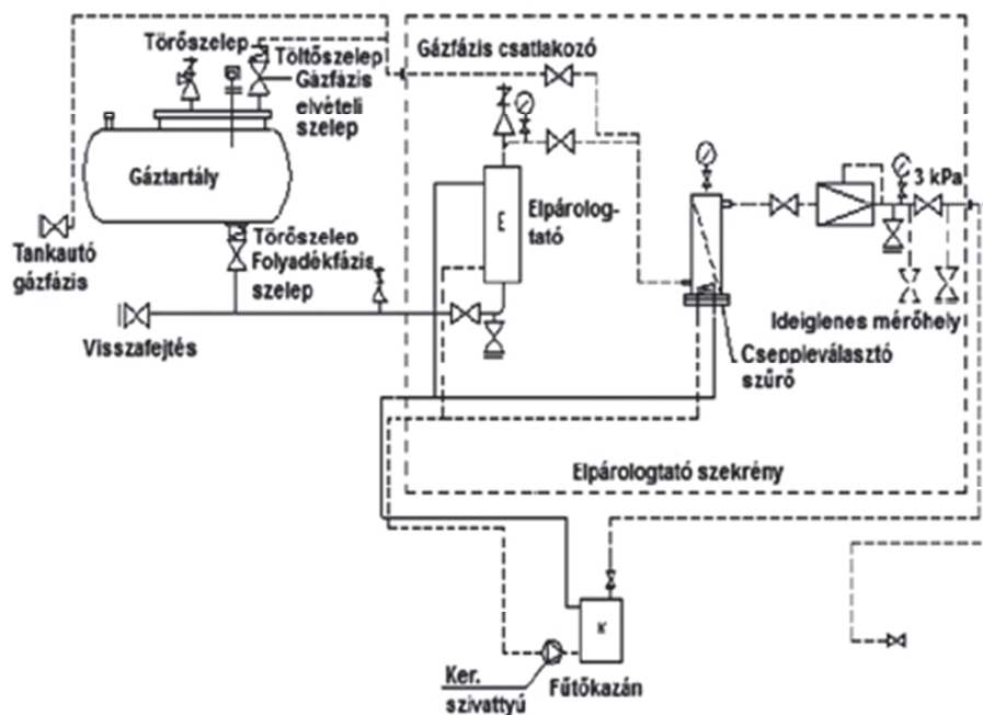
4. ábra Csatlakozóvezetékre dolgozó elpárologtató szekrényes beépítése
