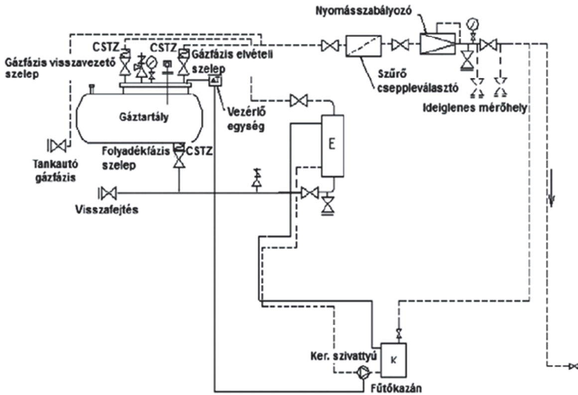
3. ábra: Tartályra dolgozó elpárolgató beépítése
