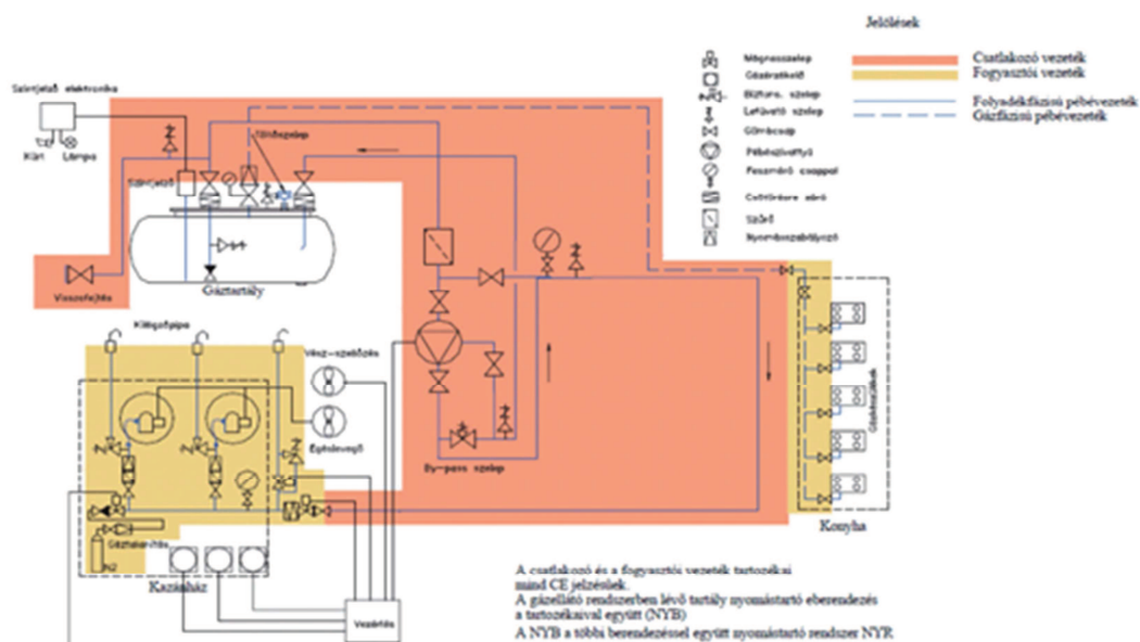
8. ábra: A csatlakozó- és a fogyasztói vezeték határai szivattyús és egyszerű PB-gáz ellátó rendszerénél
