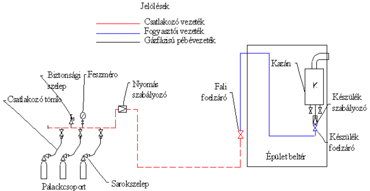
II.-12. sz. ábra Csatlakozó vezeték palackcsoportos pégégz ellátó rendszer esetén
