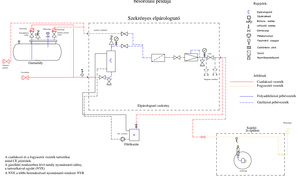
II.-10. sz. ábra A csatlakozó vezeték elpárologtató pébéégz ellátó rendszer esetén
