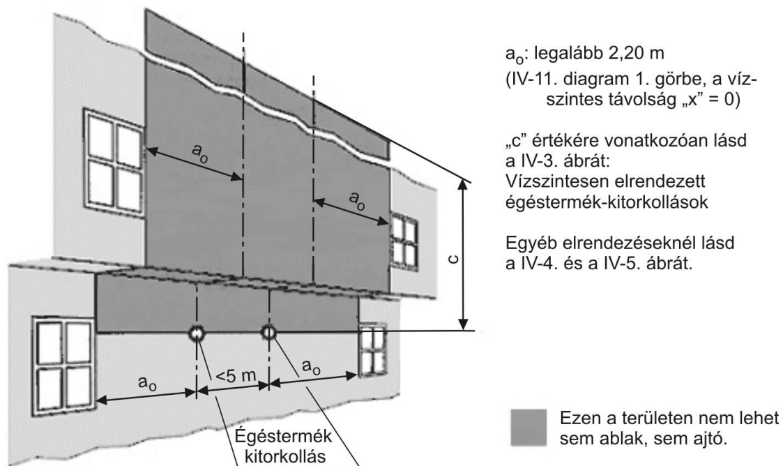
IV.-7. sz. ábra Kétszeres égéstermék-kitorkollások legkisebb távolsága nyitható ablakoktól vagy homlokzati ajtóktól előreugró homlokzatok esetén
