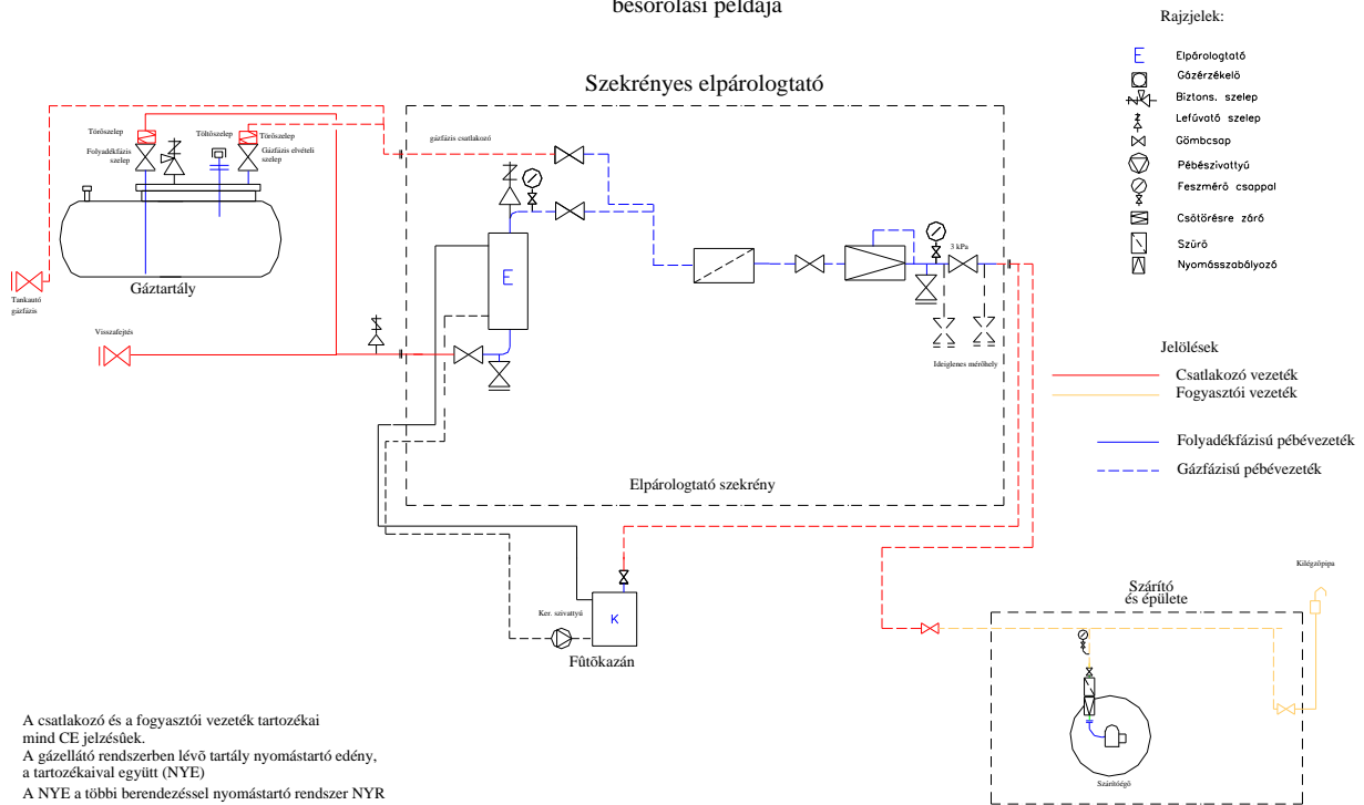
II.-10. sz. ábra A csatlakozó vezeték elpárologató pébéégáz ellátó rendszer esetén
