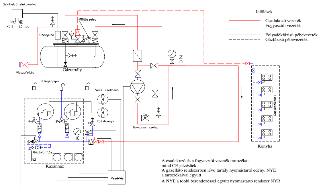
II.-11. sz. ábra A csatlakozó vezeték szivattyús pébéégáz ellátó rendszer esetén
