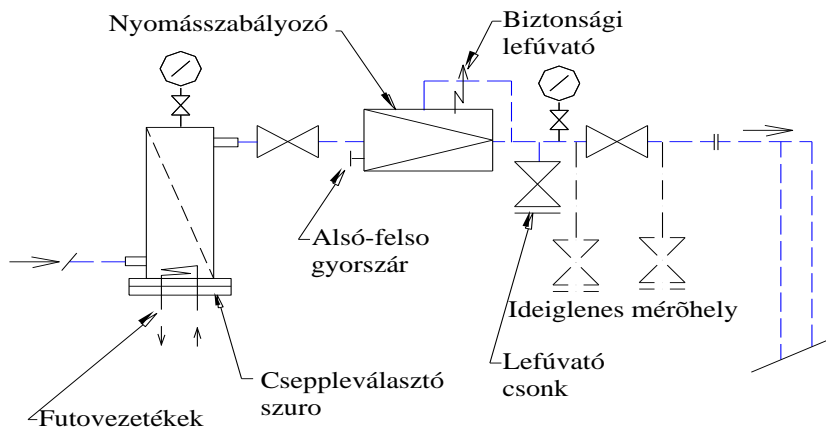
III.-9. sz. ábra Pébégáz párologtatós rendszerű nyomásszabályozó berendezés. Az ábra szerinti kialakításban a külön szűrő csepleváltató funkciót és másodlagos elpárologtatást is szolgál.
