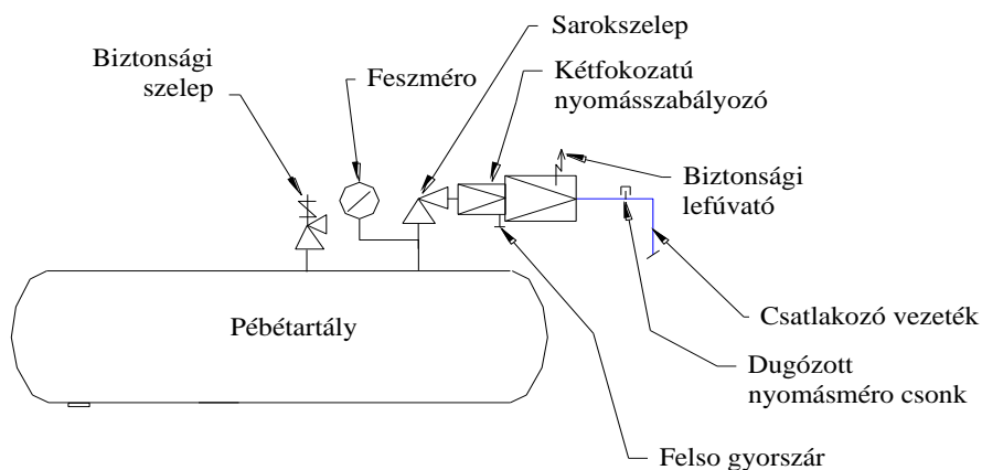
III.-8. sz. ábra Pébégáz tartályra szerelt nyomásszabályozó max. 24 [kg/h] gázéltételre
