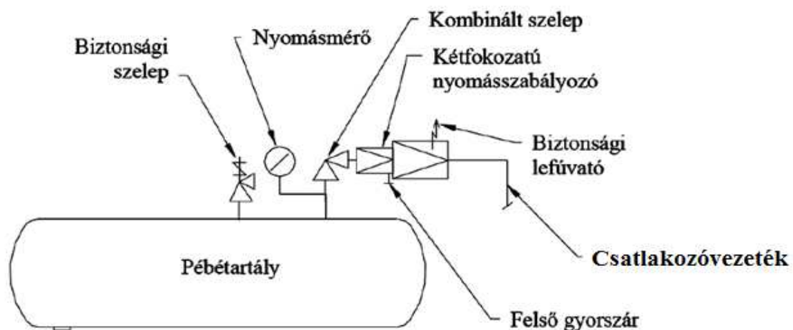
1. ábra: Tartályra szerelt nyomásszabályozó max. 24 kg/h gázelvételre
