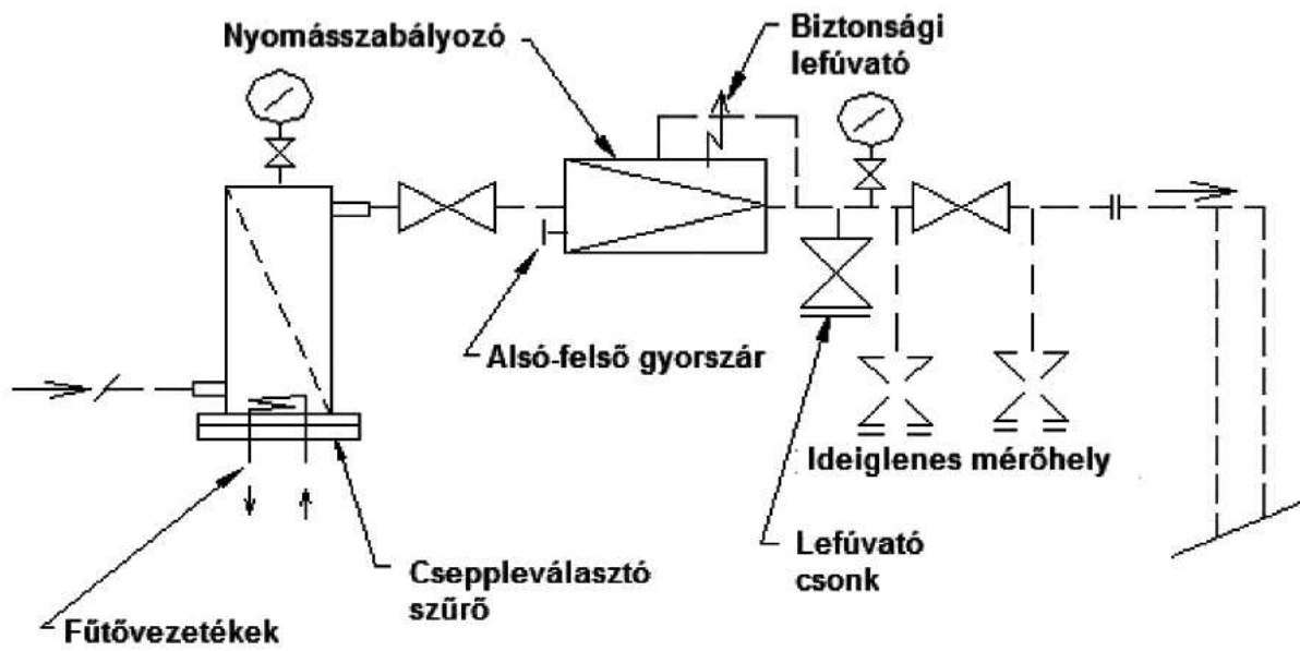
2. ábra: Párolgató rendszerű nyomásszabályozó berendezésre
