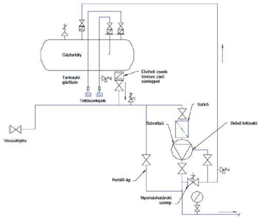
5. ábra Szivattyú alkalmazása
