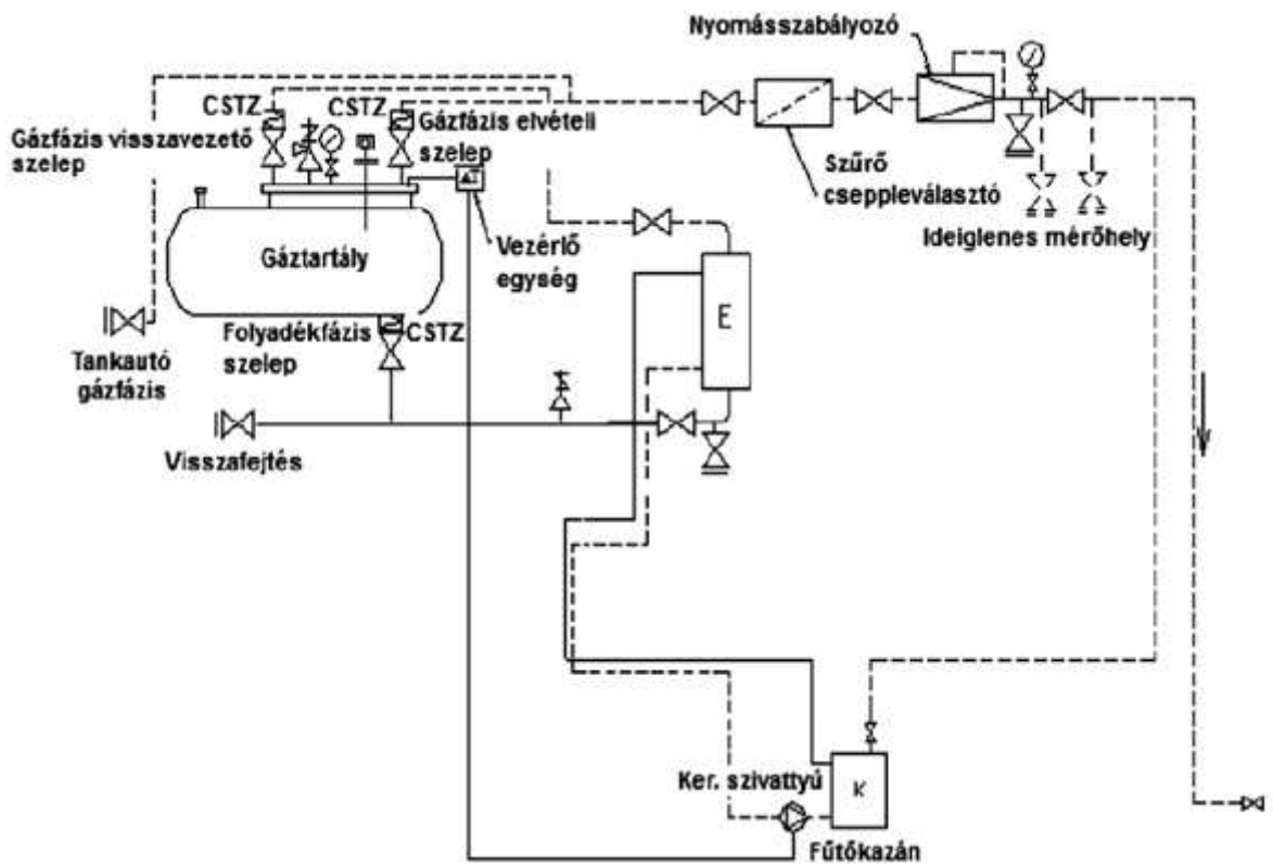
3. ábra: Tartályra dolgozó elpárolgató beépítése
