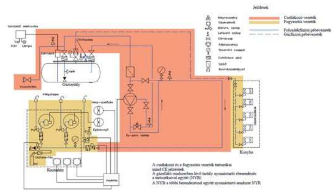
8. ábra: A csatlakozó- és a fogyasztói vezeték határai szivattyús és egyszerű PB-gáz ellátó rendszernél
