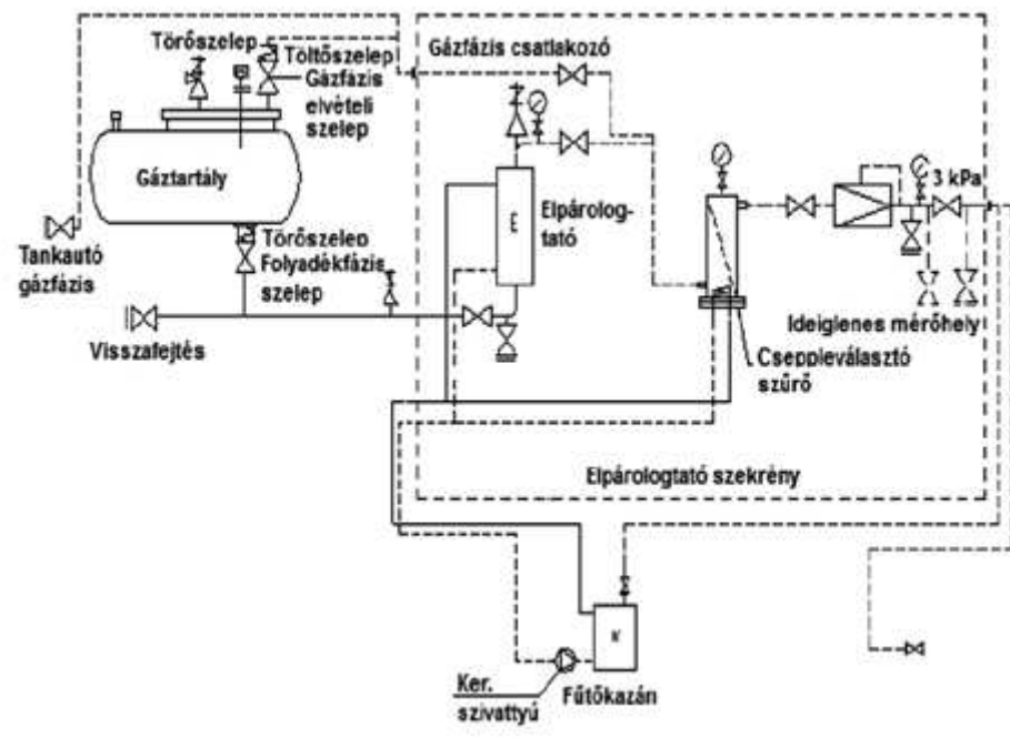
4. ábra Csatlakozóvezetékre dolgozó elpárolgató szekrényes beépítése
