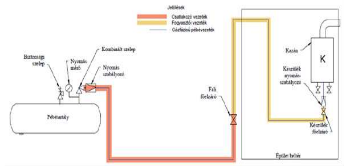
6. ábra: A csatlakozó- és a fogyasztói vezeték egyszerű PB-gáz ellátó rendszerénél
