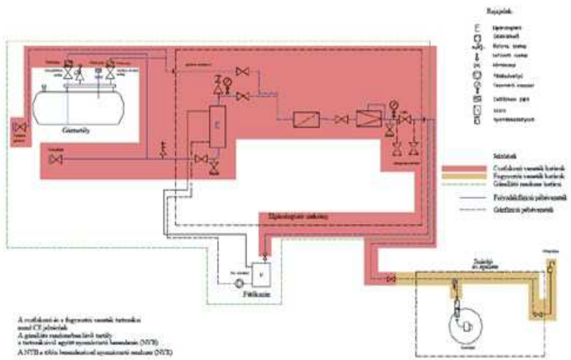
7. ábra: A csatlakozó- és a fogyasztói vezeték határai szivattyús és egyszerű PB-gáz ellátó rendszerénél
